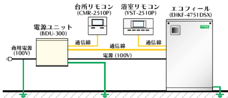
構成図
